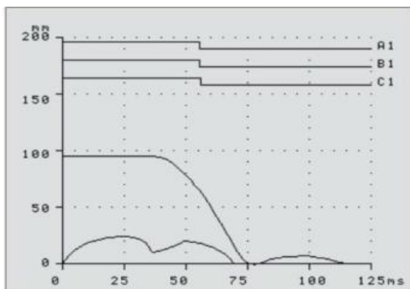
分闸测试图形
