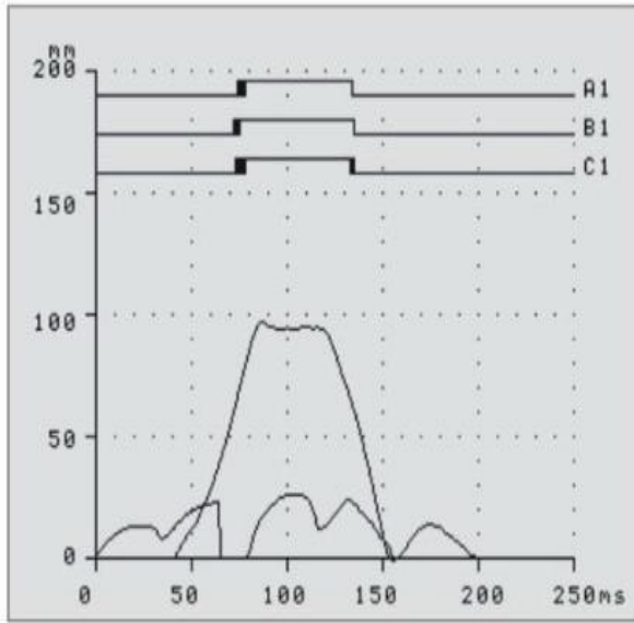
合--分闸测试图形
