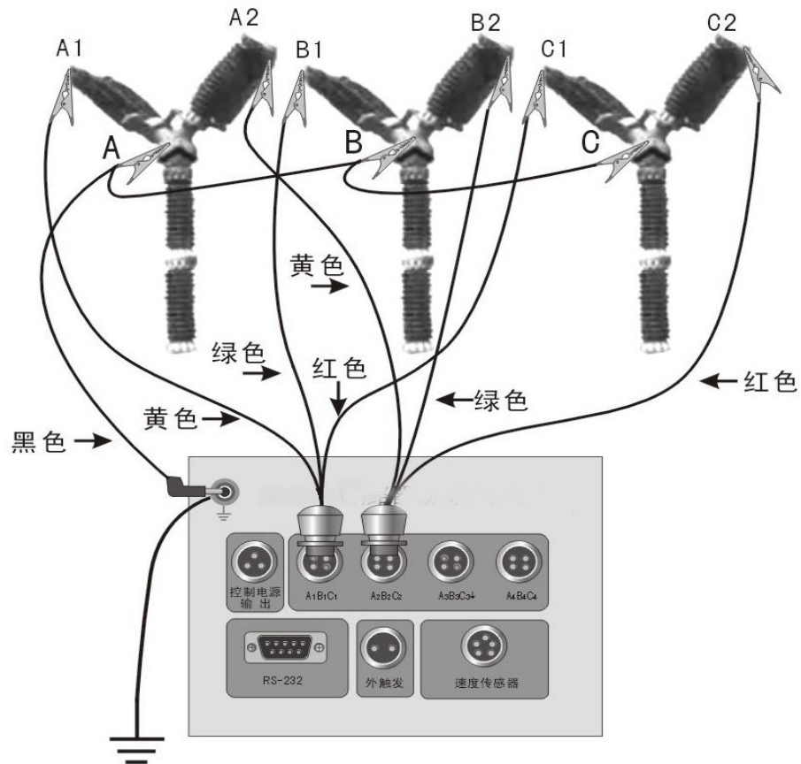
断口接线图（六断口）
