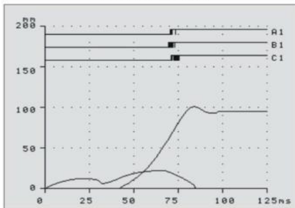
合闸测试图形
