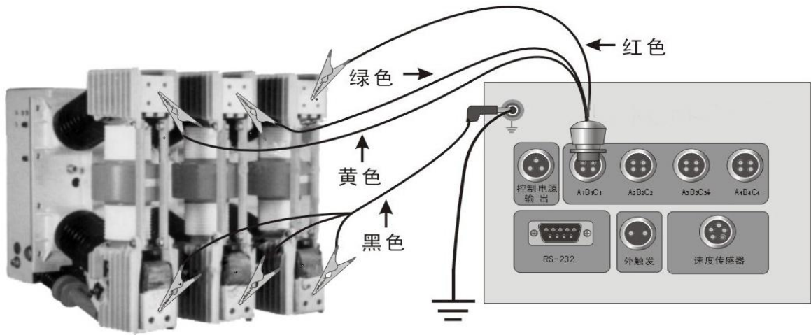
断口接线图（三断口）
